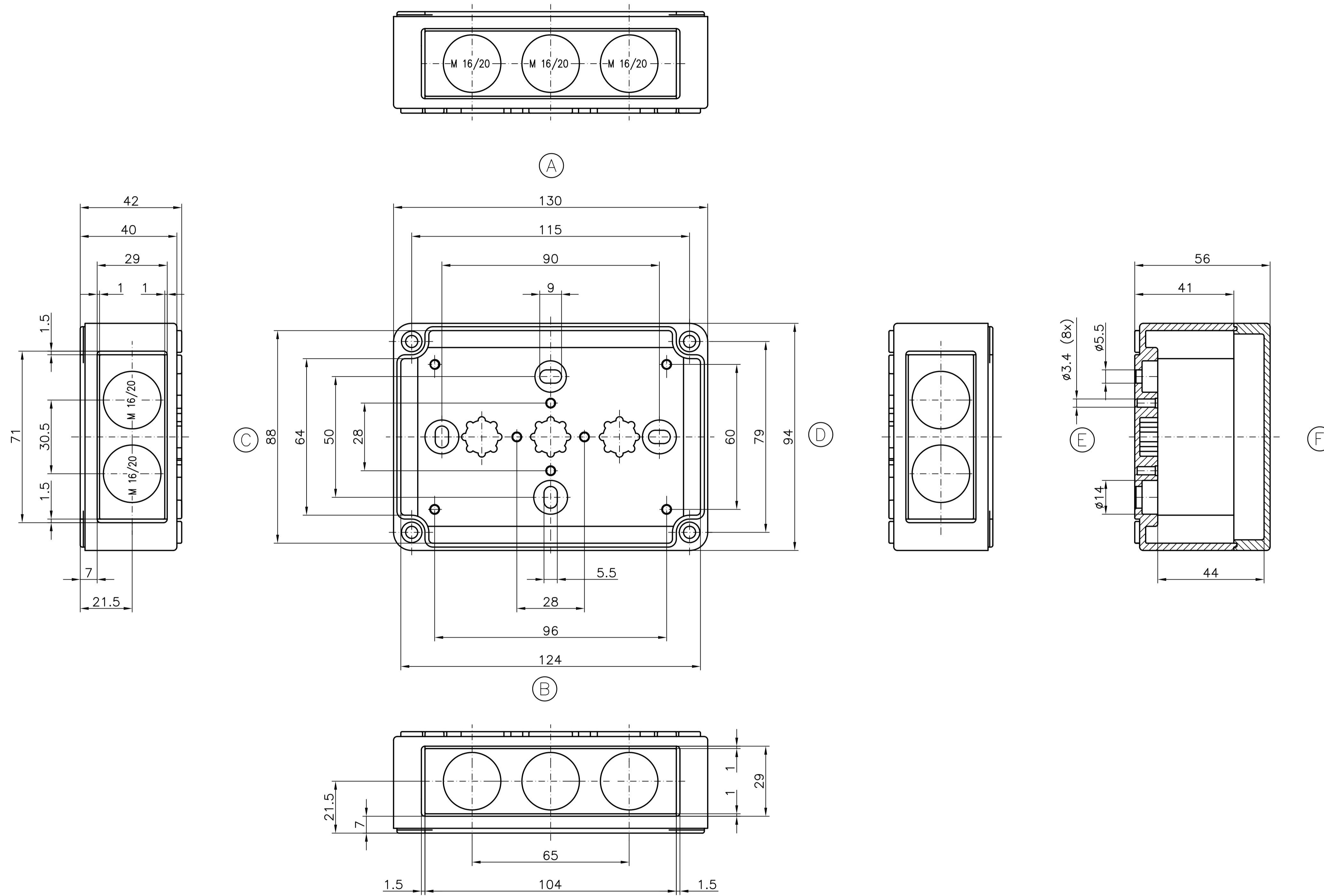
Kompaktgehäuse PCI 04-6M Bestell-Nr. 60.091315
